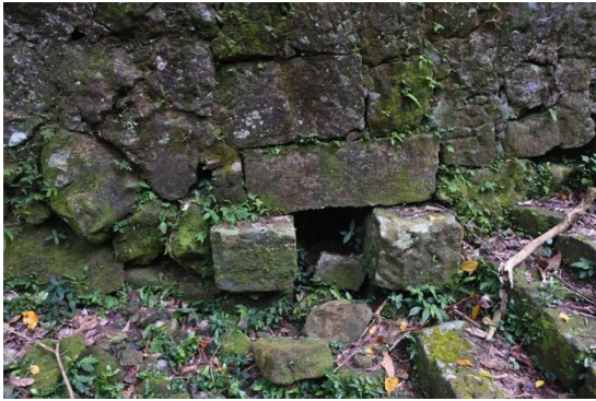
圖 3-20 谷積和平積混合砌石駁坎 (資料來源：研究團隊攝影)
